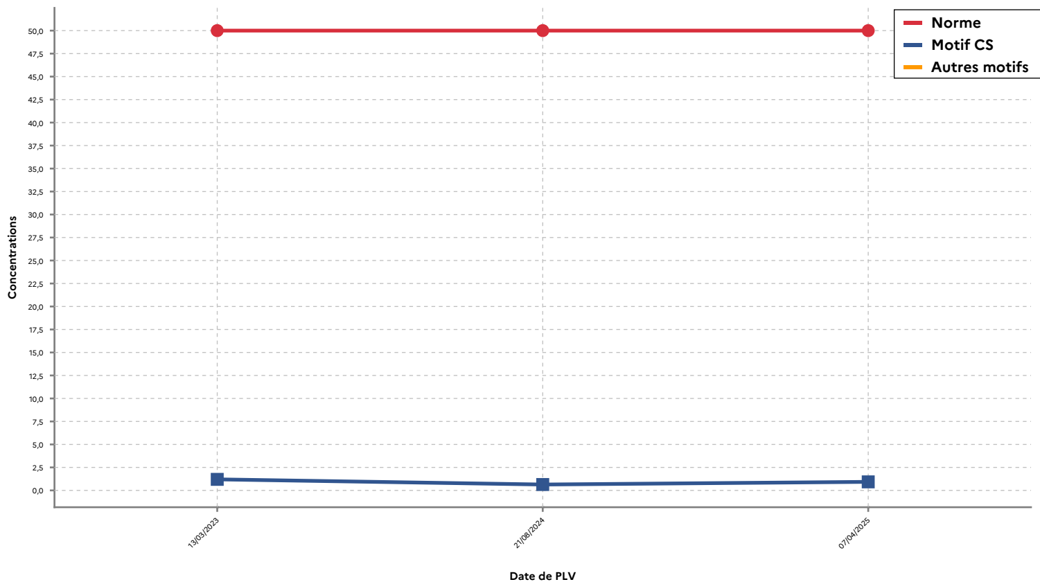
Concentration en nitrates (mg/L) sur 3 ans pour le captage/mélange de captage 012000010 - LE SARLENQ
